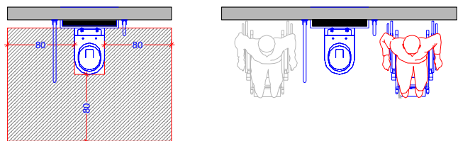
FIGURA 4 – Sono riportati, a titolo esemplificativo, diversi tipi di accostamento al sanitario che prevedono il trasferimento dalla carrozzina allo stesso (tazza wc e seggiolino doccia) con i relativi spazi di manovra.
